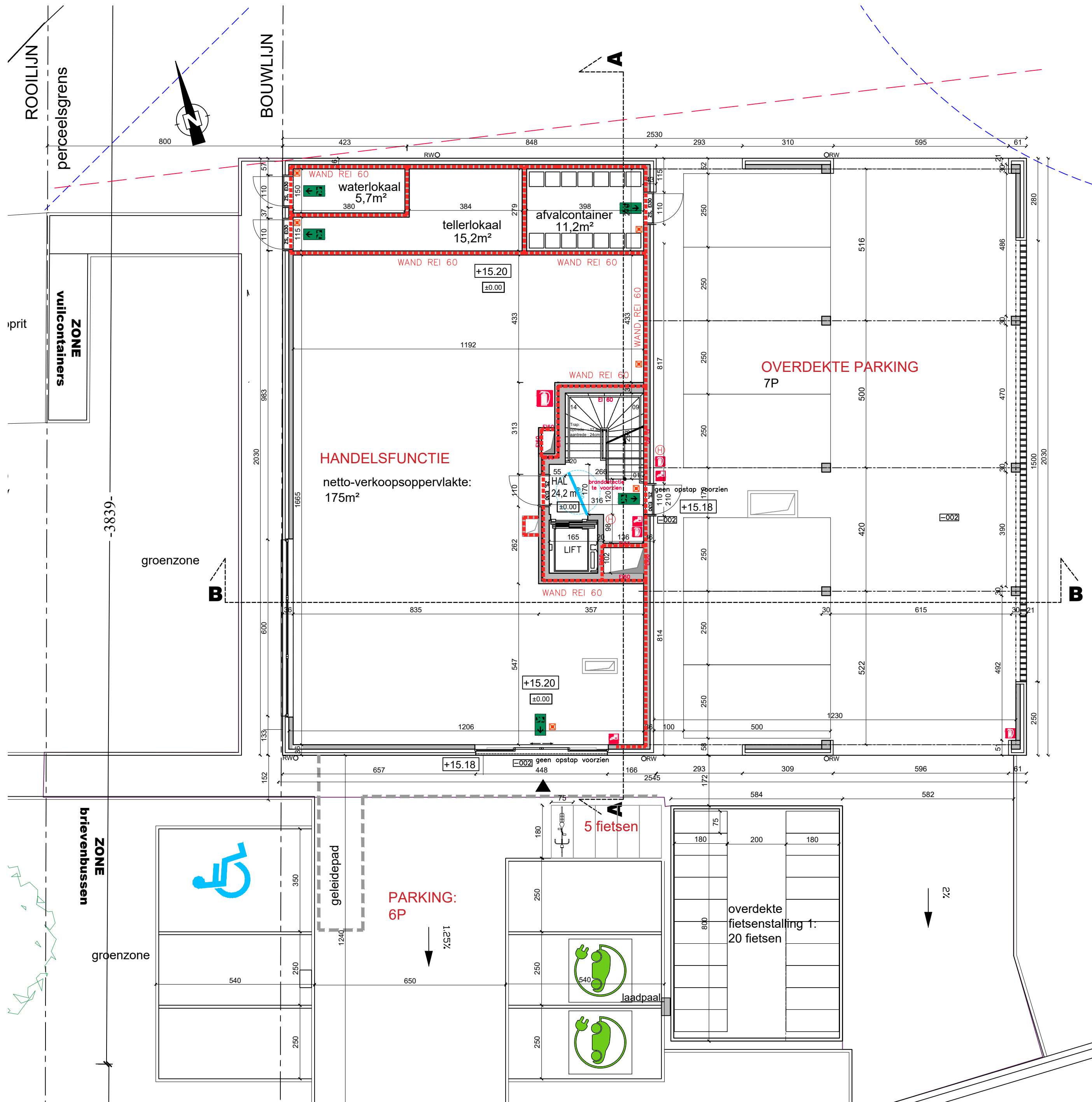
GELIJKVLOERS - MEERGEZINSWONING + HANDEL NIEUWE TOESTAND SCHAAL: 1/100
